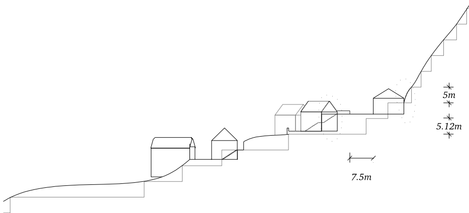
Fig 22. Seccion pera urbanizacion n o 2, diferéncia de còta.
