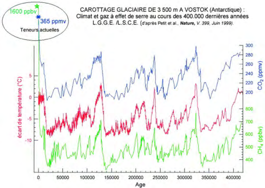
Fig. 7: Esquèma gessut deth testimòni de Vostok enes gèus der Antartic mostrant es variacions climatiques des de 420 000 ans correlacionadi damb es emissions de gas coma efèctes ivernacle. Se ve qu'eth Darrèr Maximum Glacièr (DMG) se passèc hè 22 000 ans apruprèt, periòde dera cultura des Solutrens. Er anterior tàs 140 000 ans.
